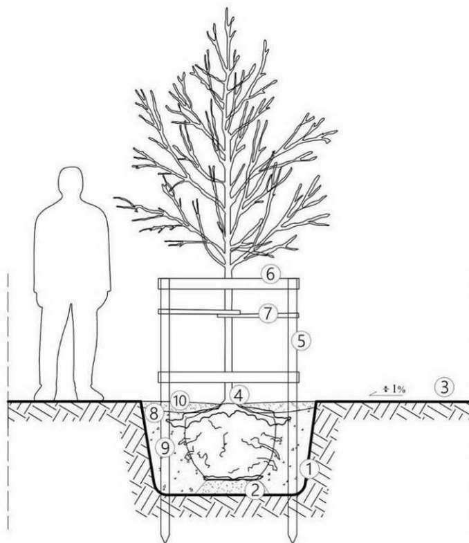
Ryc. 33. Schemat sadzenia drzewa (wariant 1) w warunkach sprzyjających (drzewo o wymiarach 12-14cm i wys. 200cm stabilizowane za pomocą 3 niskich palików) (oprac. Ł. Dworniczak, M. Kulon).
