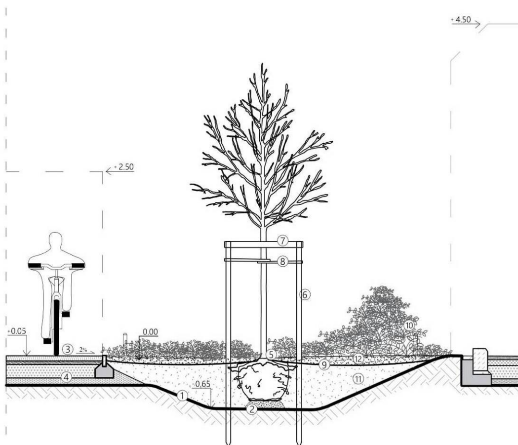
Ryc. 34. Schemat sadzenia drzewa (wariant 2) w pasie drogowym – w trudnych warunkach. Przedstawiono drzewo o wymiarach 16-18 cm i wys. 400 cm stabilizowane za pomocą 3 niskich palików (oprac. Ł. Dworniczak, M. Kulon).
