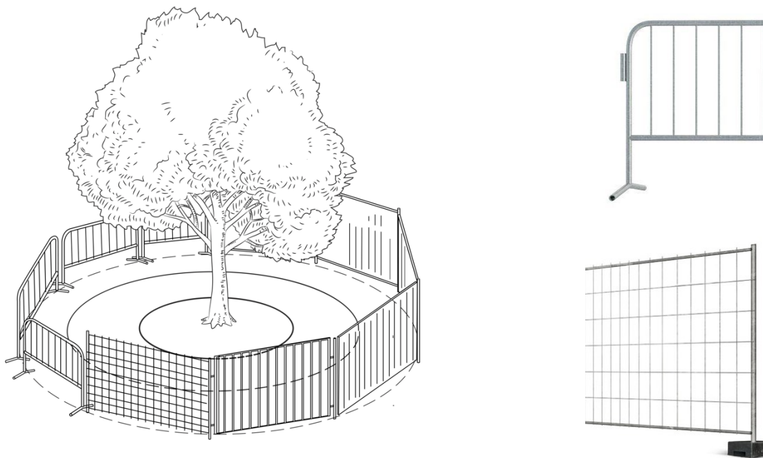
Ryc. 6. Schemat tymczasowego wyгородzenia strefy ochrony drzewa oraz przegląd wyгородzeń mobilnych.
